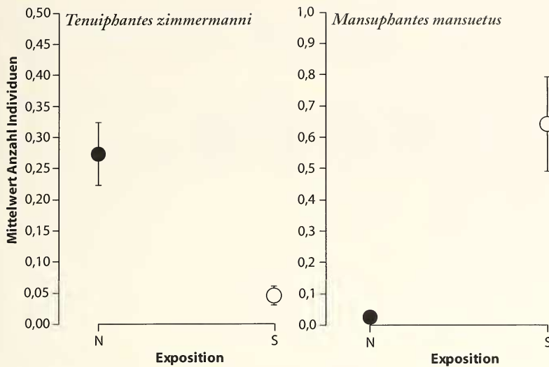
Abb. 9: Mittelwert (±SE) der erfassten Anzahl Individuen zweier Arten pro Falle und Periode. Vergleich der Hangexposition. (●= Nordhänge; ○= Südhänge).
